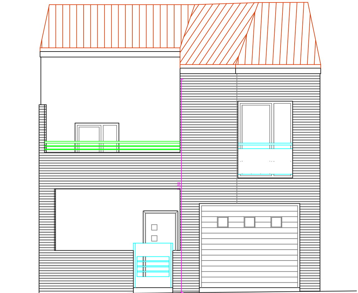
alzado A1-A1'
